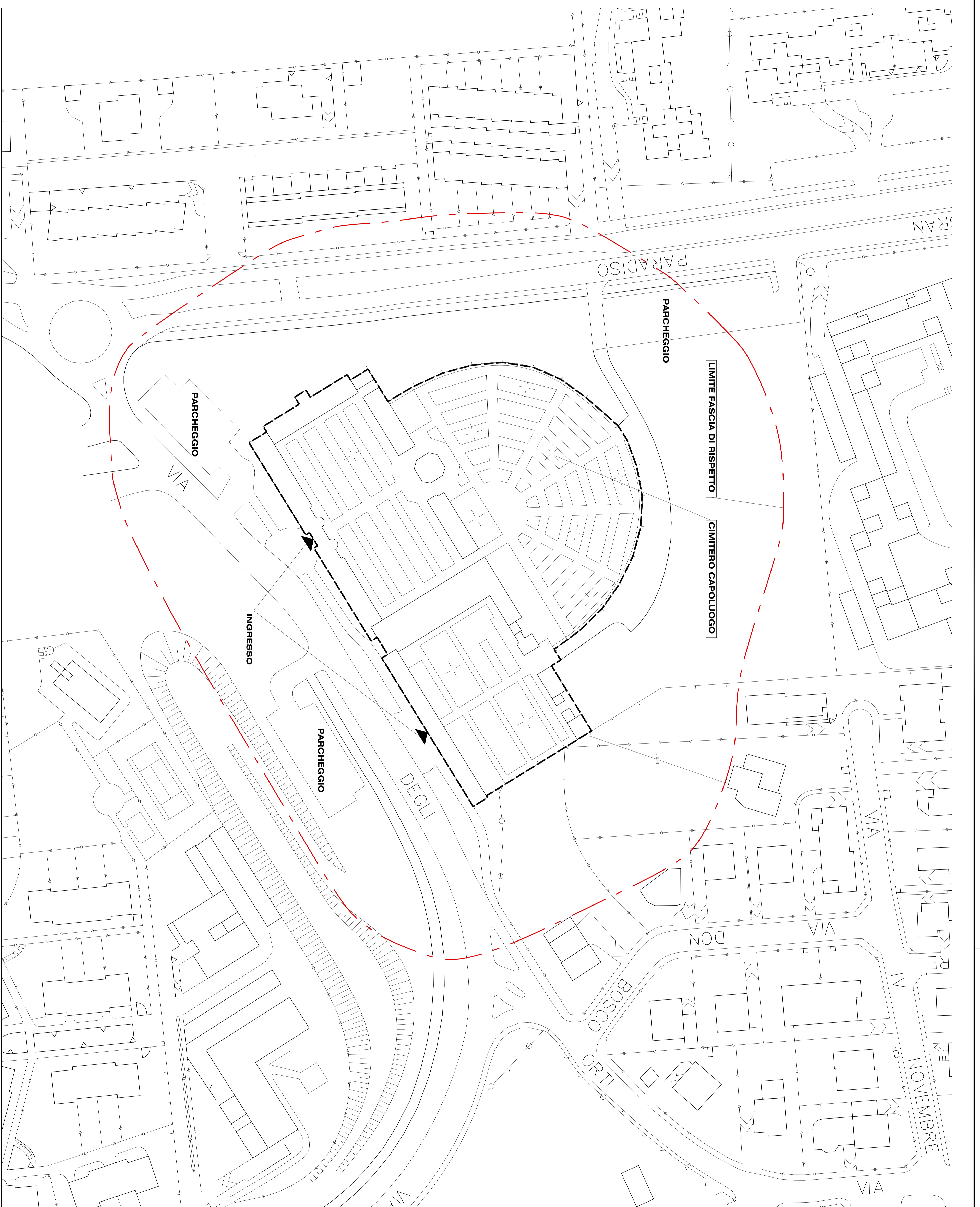
PLANIMETRIA DEL CIMITERO CAPOLUOGO - SCALA 1:500
